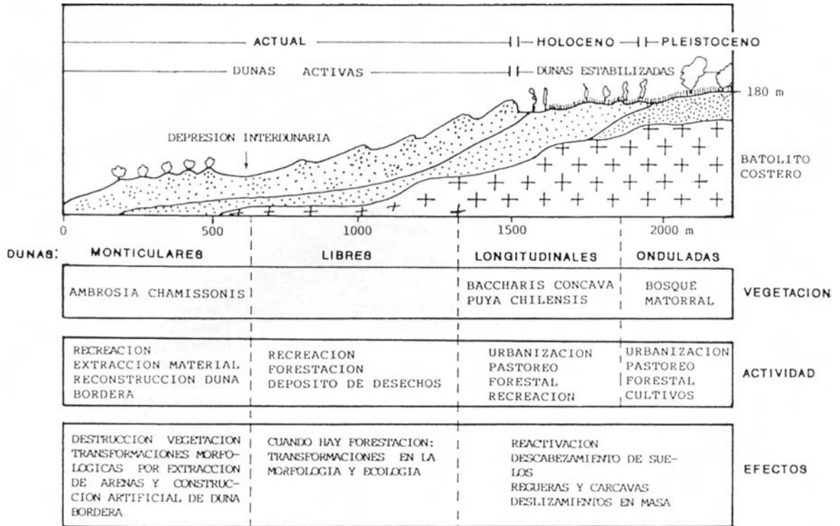
Fig. 1. Tipología de geoformas dunarias en Chile. Principales actividades humanas y sus efectos. Typology of Dune geomorphs in Chile. Principal human activities and their effects.
